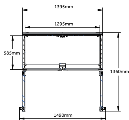
Вид сверху
