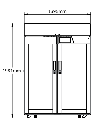
Вид спереди
